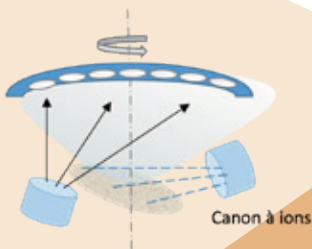
Figure 4 : Schéma de principe (à gauche) du procédé de pulvérisation par faisceau d'ions avec assistance ionique (DIBS, Dual Ion Beam Deposition ), et photographie (à droite) de l'intérieur d'une machine fonctionnant sur ce principe à l'Institut Fresnel- 2000. Photo © Institut Fresnel
